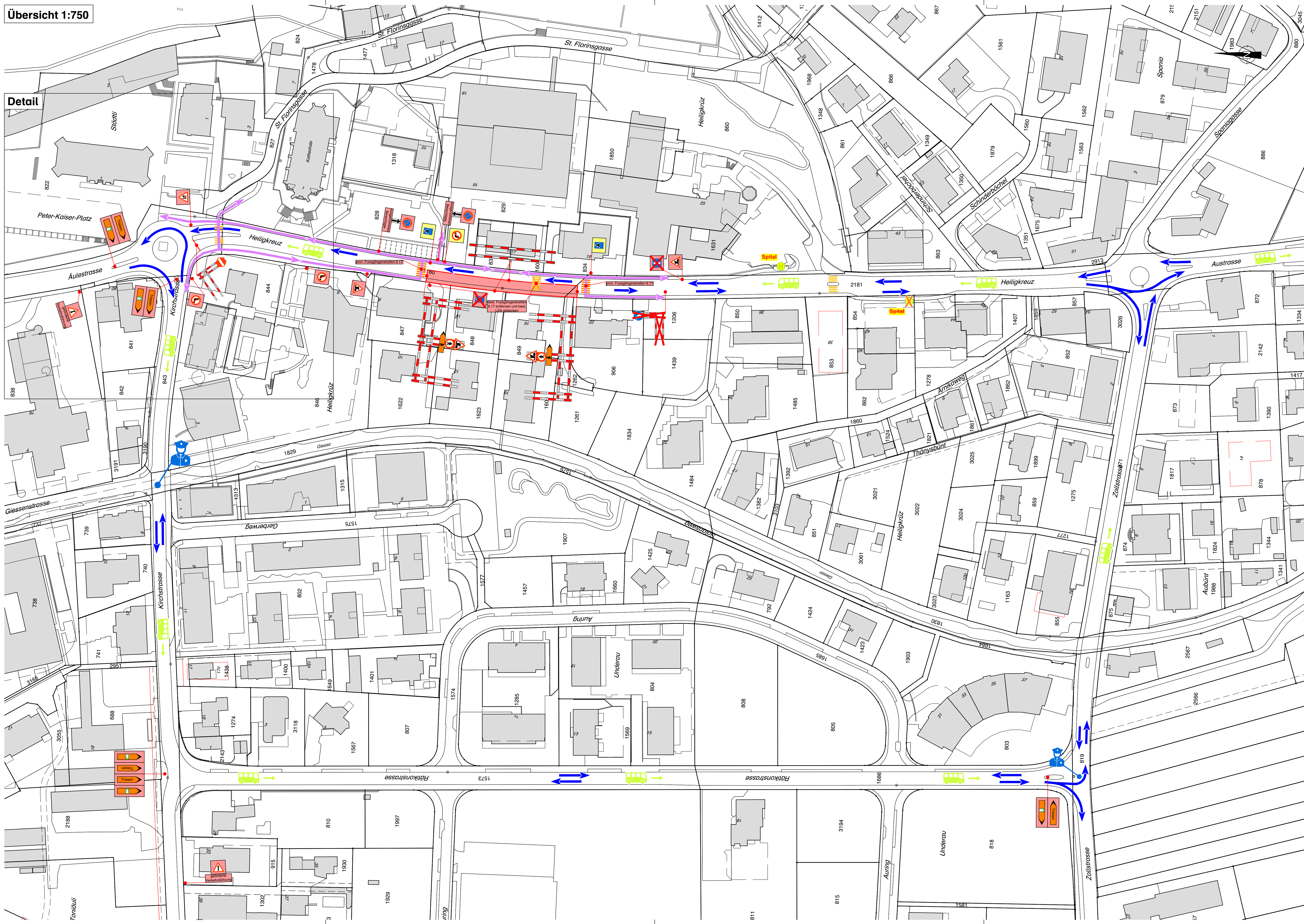
Detail Kreisel Heiligkreuz - Aulestrasse - Kirchstrasse 1:500
